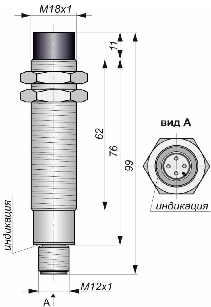
Габаритный чертеж
